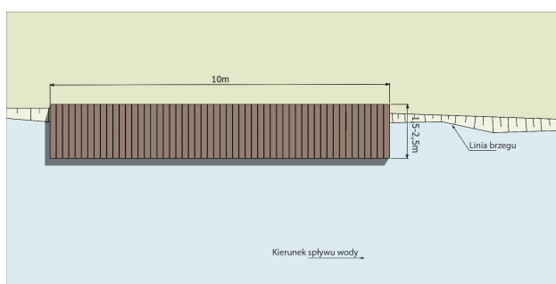
Il. 1. Schemat - Pomost równoległy do nurtu mocno utwierdzony w terenie
