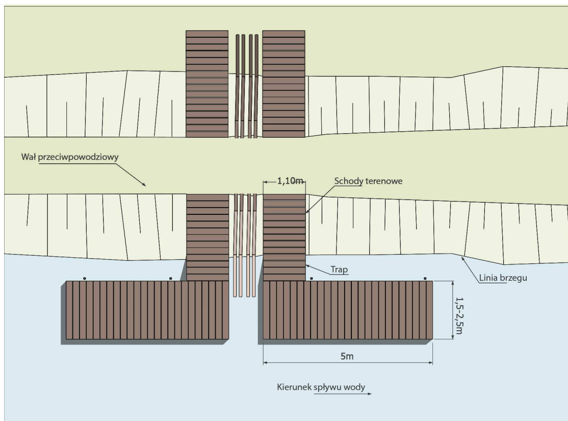
Il. 15. Schemat - Pomost pływający równoległy do nurtu, schody obustronnie
